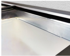
■ Duvar Profili Üst Conta Detayı Wall Profile Upper Gasket Detail
