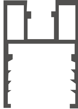
BAZA DİKEY PLINTH VERTICAL Stok : 6 mt 7 mt Ağırlık / Weight: 0,616 Kg/m
