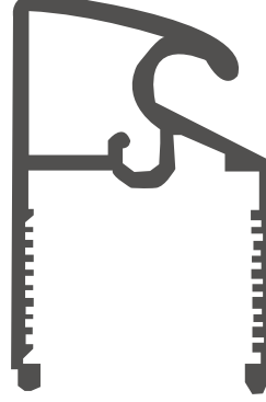
ÜST KÜPEŞTE BAĞLANTI PROFİLİ MEDIUM GLA UPPER HANDRUFF CONNECTION PROFILE SS PROFILE Stok : 6 mt 7 mt Ağırlık / Weight: 0,600 Kg/m
