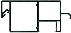
İkili Kutulu Kanat Üst Kenet Twin-Box Wing Upper Brace
