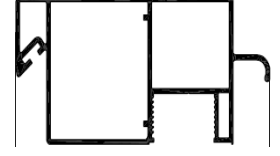
2'Lİ KANAT ÜST KENET 2-WING UPPER CLAMP
