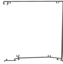
ŞASE CHASSIS Stok : 7 mt Ağırlık / Weight: 2,263 Kg/m
