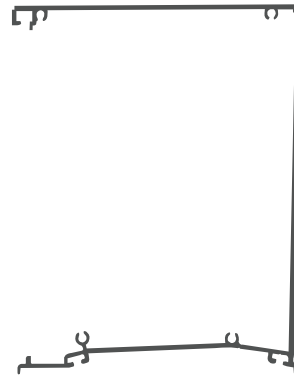
ŞASE CHASSIS Stok 6 mt 7 mt Ağırlık / Weight: 2,263 Kg/m
