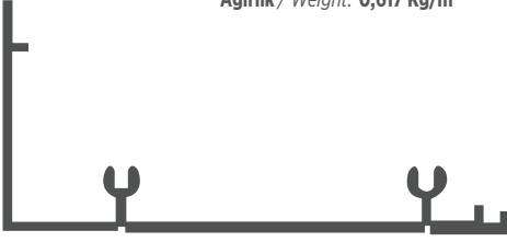
ÜST İÇ KAPAK TOP INNER COVER Stok 6 mt 7 mt Ağırlık / Weight: 0,617 Kg/m
