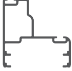
ISICAM 45° KÖŞE THERMOPANE 45° CORNER
