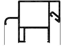
KANAT ÜST KENETİ WING UPPER CLAMP
