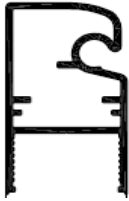
TİJLİ ÜST KÜPEŞTE UPPER RAILING WITH BARS Stok : 7 mt Ağırlık / Weight: 0,693 Kg/m
