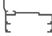
ISICAM KÜÇÜK "H" THERMOPANE SMALL "H"
