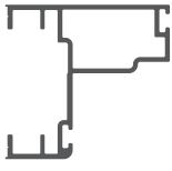
ISICAM 45° KÖŞE THERMOPANE 45° CORNER
